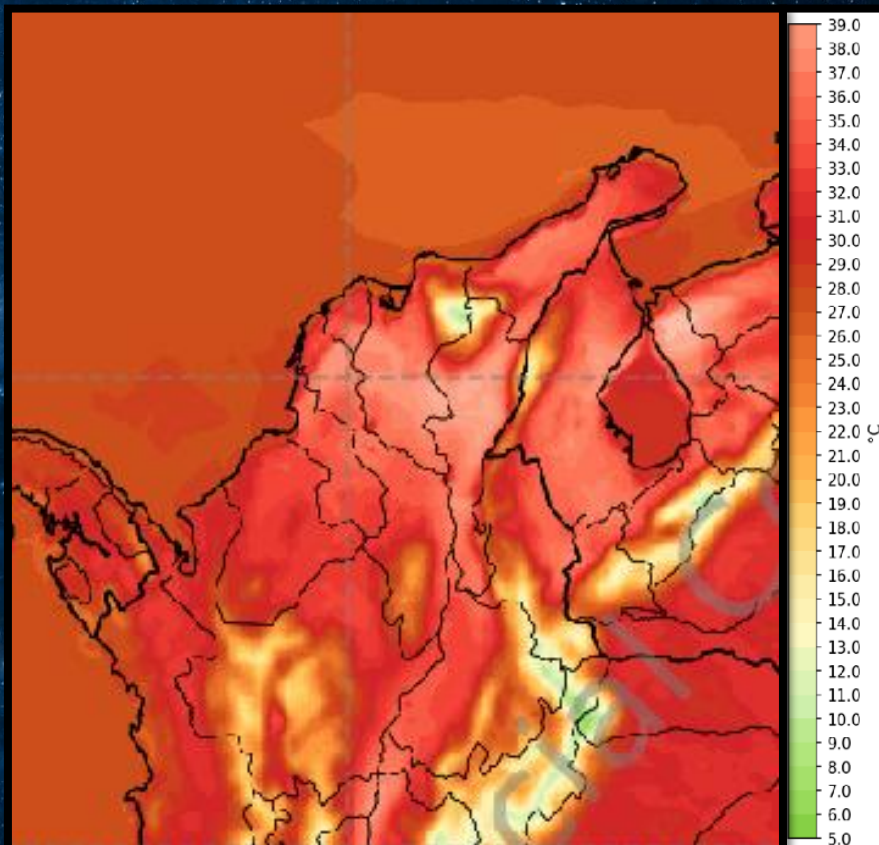
Figura 1. Tomada del Sistema de Información Meteorológica de la Fuerza Aeroespacial Colombiana (SIMFAC), la paleta de colores situado a mano derecha, describe la temperatura en grados Celsius (C°) pronosticada en la imagen, siendo la parte inferior temperaturas bajas o frías, y la parte superior temperaturas altas o calientes.
