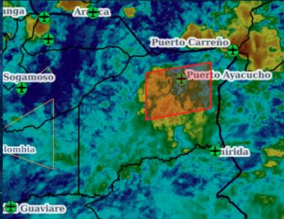
Figura 1. Imagen SAT IR 1940UTC - Tomada de Sistema de Información Meteorológica de la Fuerza Aeroespacial Colombiana (SIMFAC).
